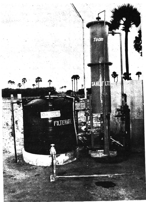
இராமநாதபுரம் மாவட்டத்தில் உவர்நீரைக் குடிநீராக மாற்றும் கருவி.
