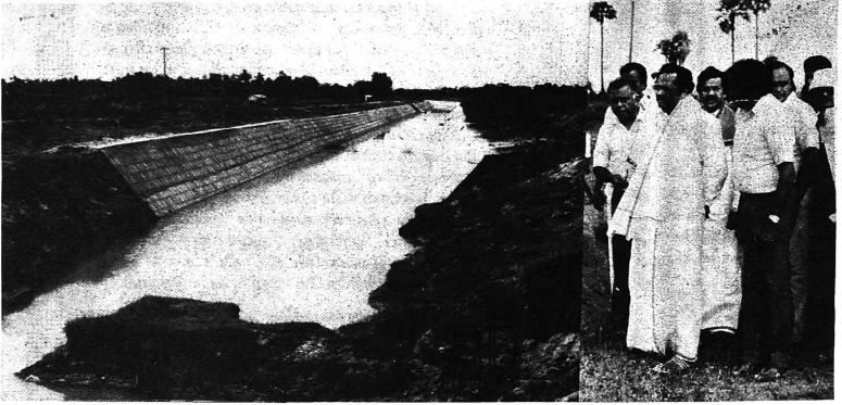
சோம சீலா அணைக்கட்டிலிருந்து பூண்டி நீர்த்தேக்கம் வரை அமைக்கப்பட்டு வரும் கால்வாயின் தோற்றம்.
