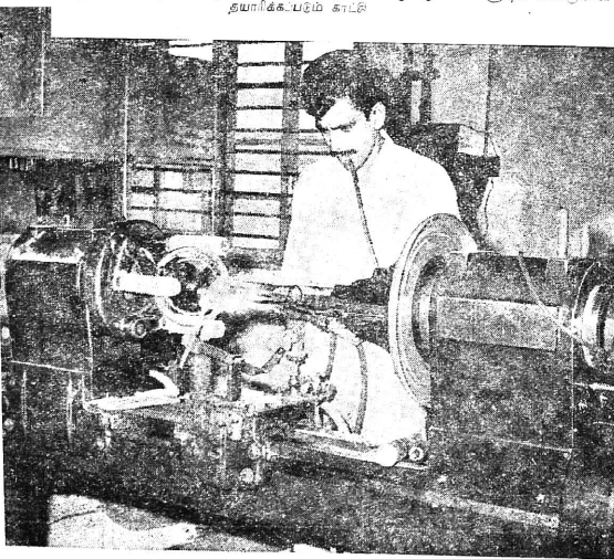
கிரோசின் வாயுவின் உதவியுடனும் வாயுவில் ஊதுவதின் மூலமும் கண்ணாடிப் பொருட்கள் தயாரிக்கப்படும் காட்சி
