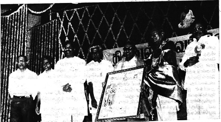
அறிஞர்களுக்கு விருது வழங்குவதில் நான் பெருமை அடைகிறேன்
