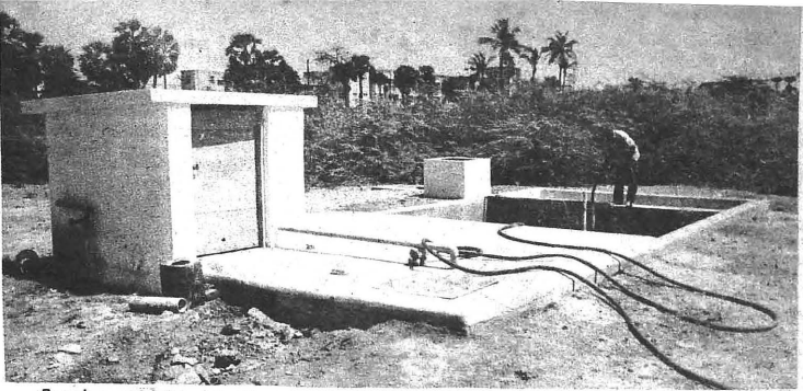
நீரைக் காய்ச்சி நன்னீர் வடித்தெடுக்கப் பயன்படும் சூரிய வெப்பத்தால் இயங்கும் கருவி.
