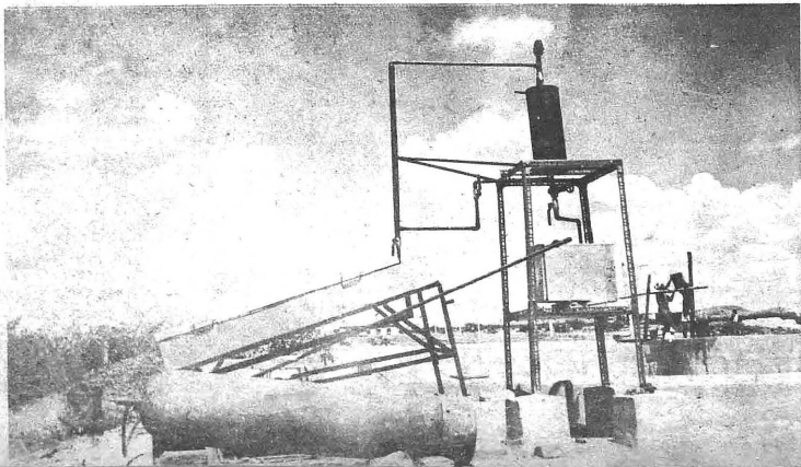
சூரிய வெப்பத்தால் இயங்கும் குளிர் சாதனம்
