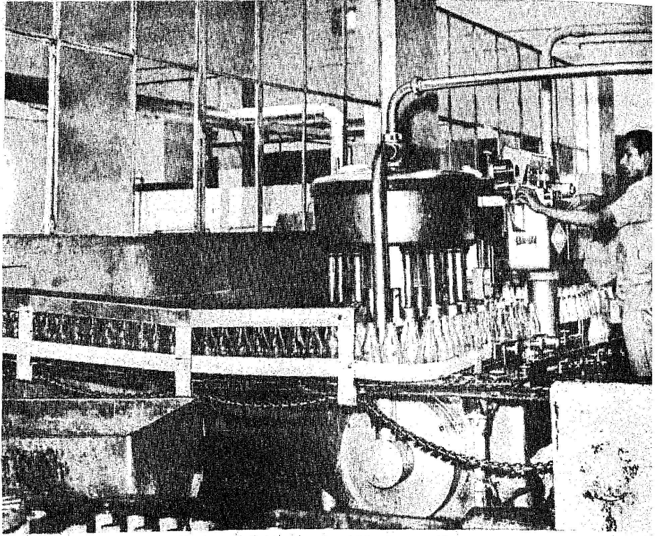
புட்டிகளில் பால் நிரப்பும் இயந்திரம்.
