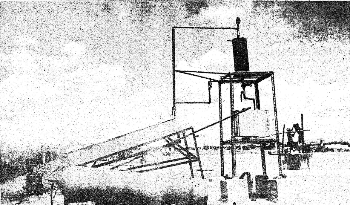
சூரிய வெப்பத்தால் இயங்கும் குளிர் சாதனம்
