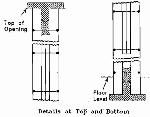
Collapsible steel door
