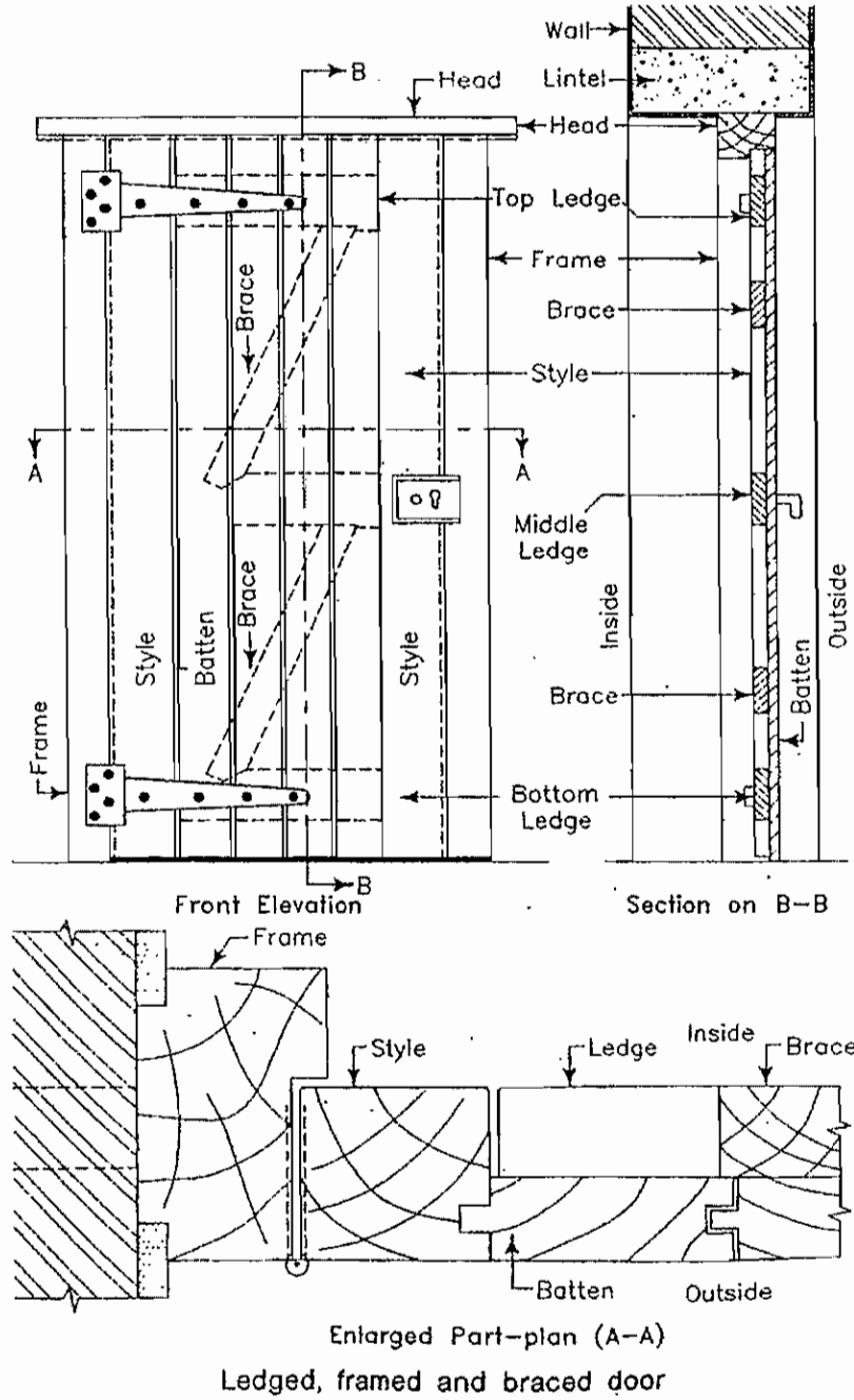
படம் 6.3.6. குறுக்குக் கட்டைகளும், சாய்வுக் கட்டைகளும், சட்டங்களும் உள்ள கதவு
