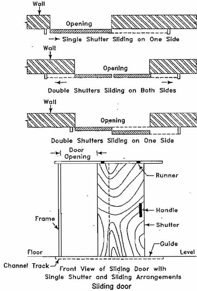
படம் 6.3.15. ஸ்லைடிங் கதவு
