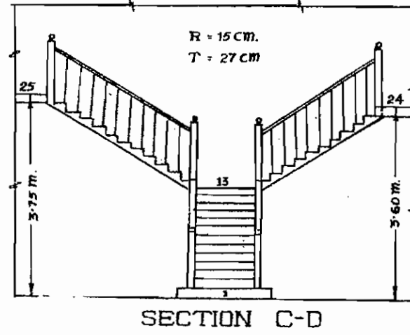
படம் 7.1.6. இரண்டாக பிரியும் படிக்கல்
