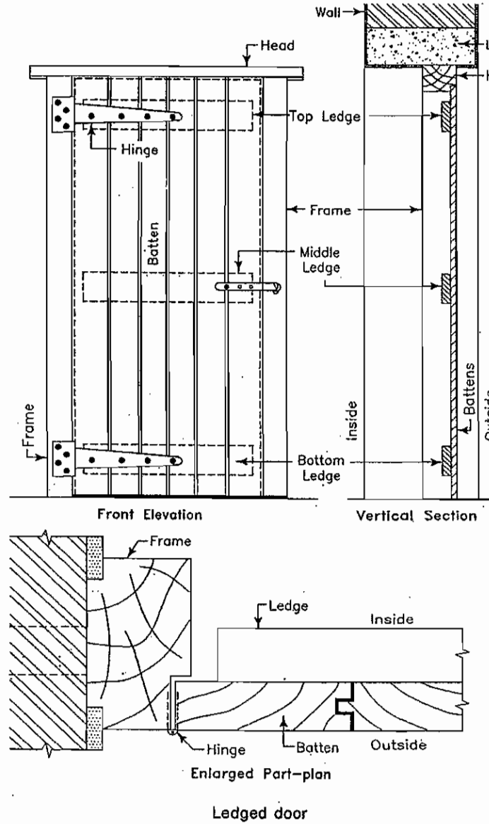
படம் 6.3.3. குறுக்குக் கட்டைகள் உள்ள கதவு
