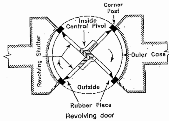
படம் 6.3.13. சுழற்கதவு
