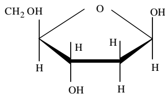
\beta -D-deoxyribose
