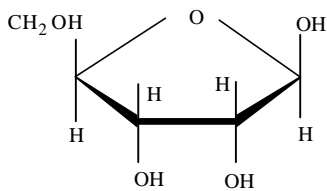
\beta -D-Ribose
