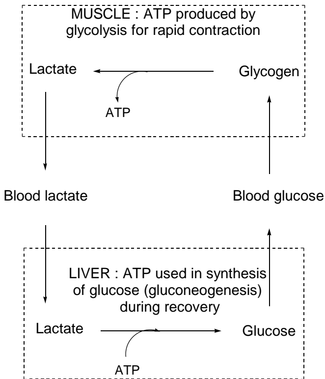
Fig. 3.6 Cori cycle
