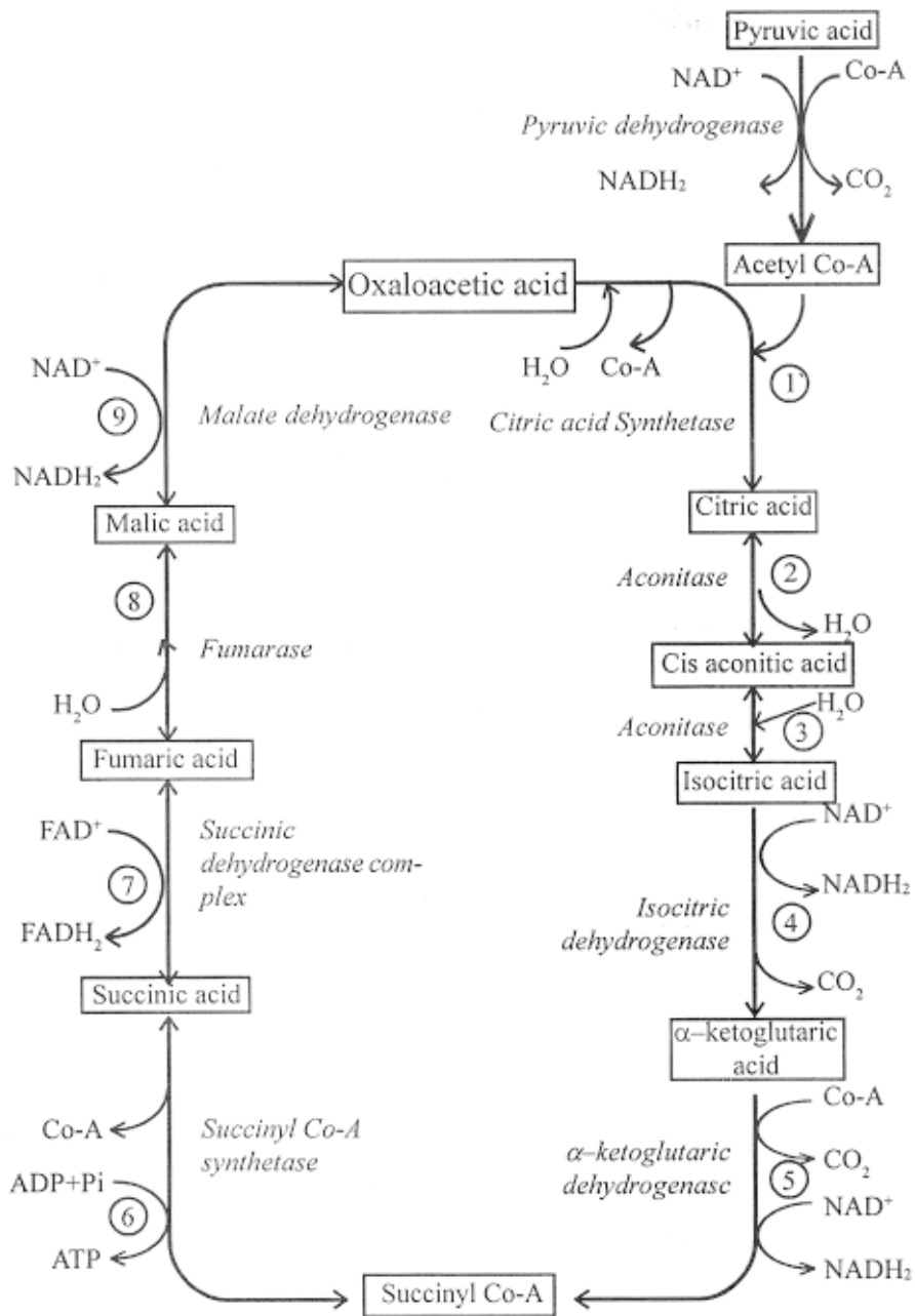
Fig. 5.15 Krebs cycle
