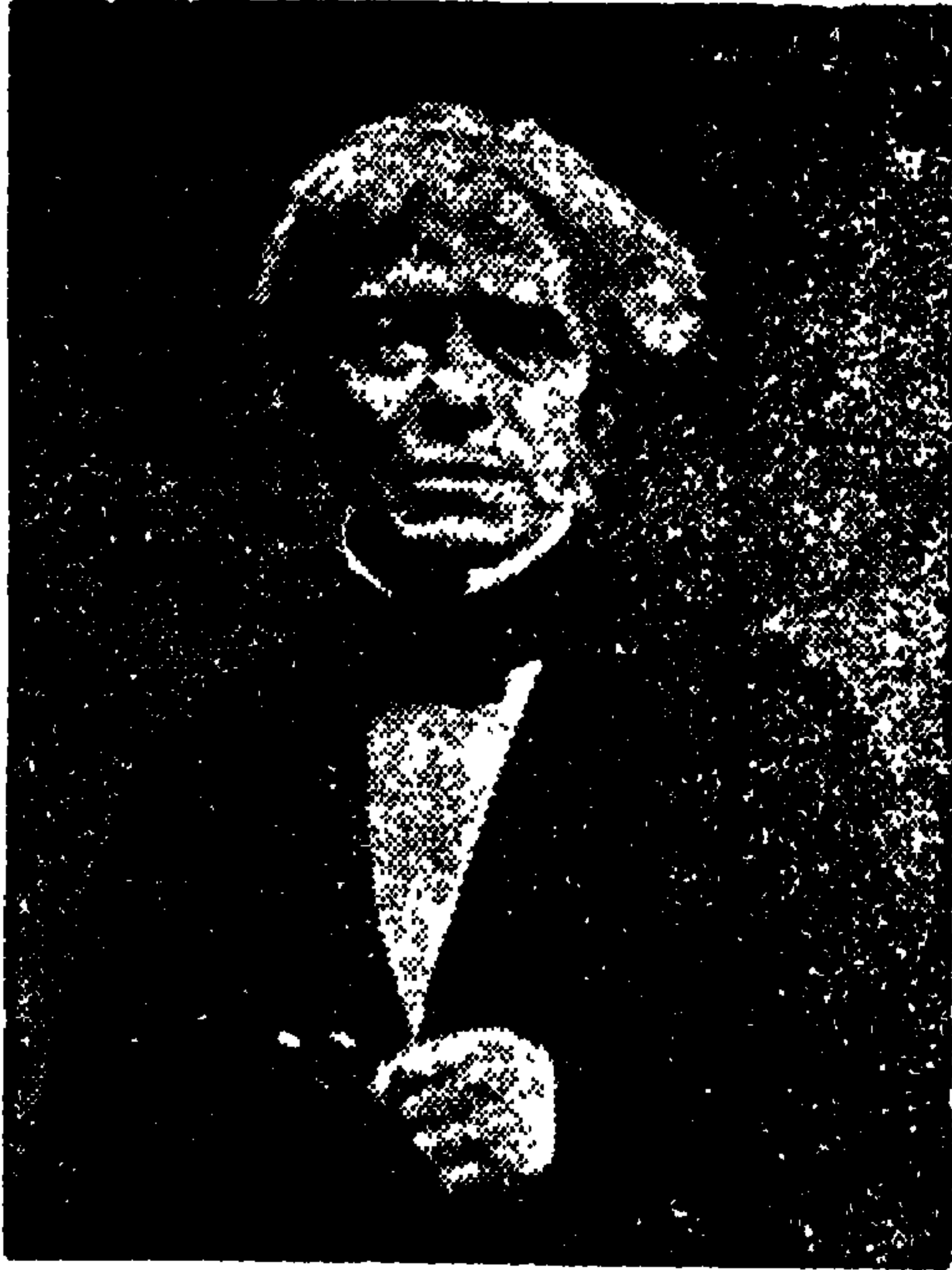
பாரடே
