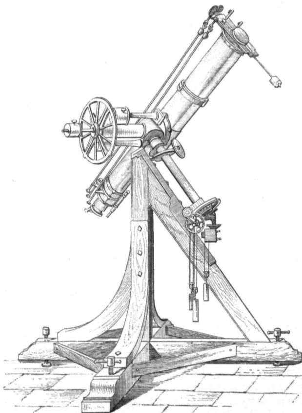
FIG. 92.—Heliumeter.
