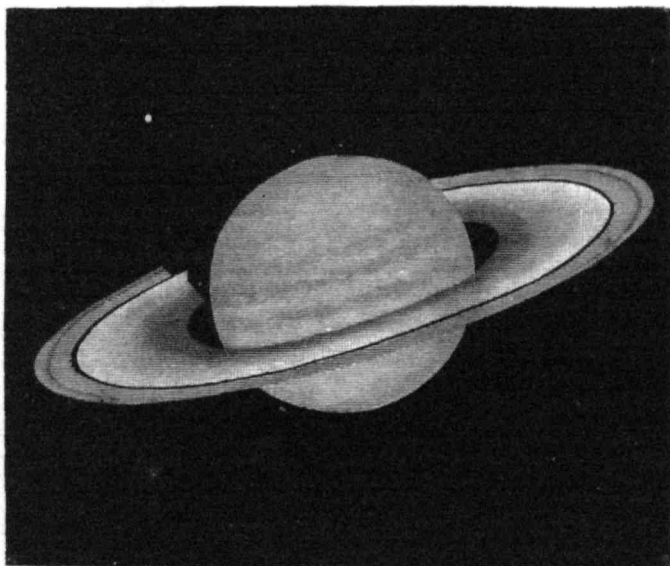
FIG. 81.—Saturn.
