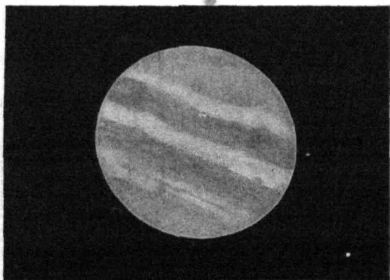
FIG. 72.—Jupiter.
