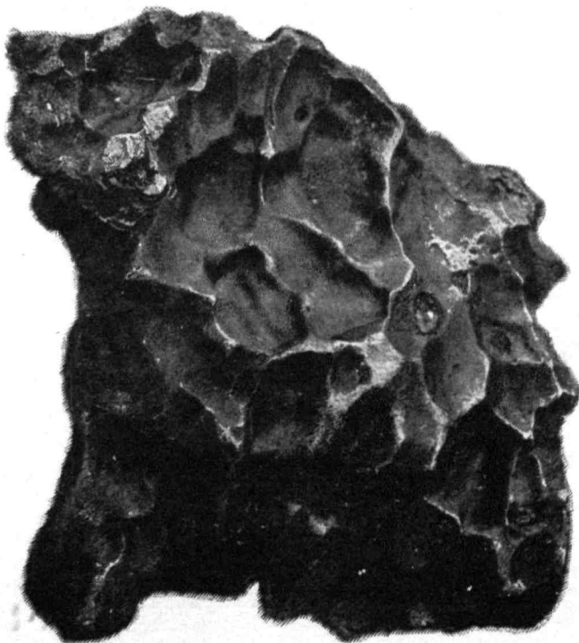
FIG. 95.—Meteorite.
