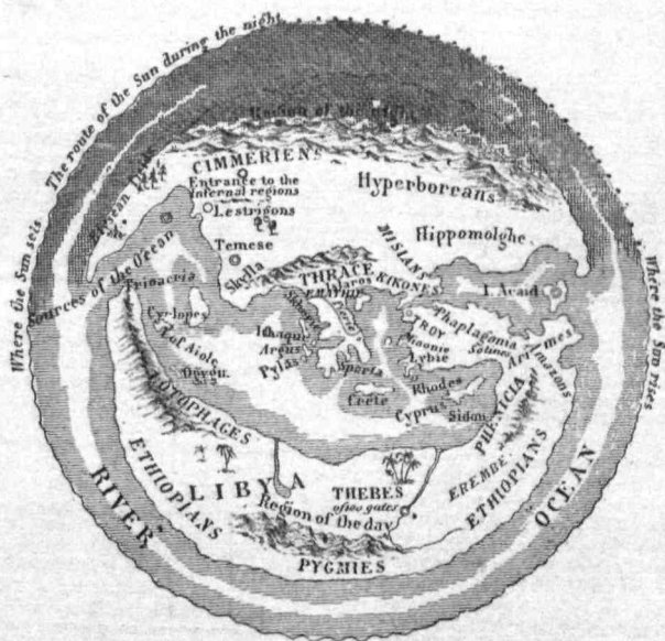
FIG. 4.—Homeric Cosmogony.
