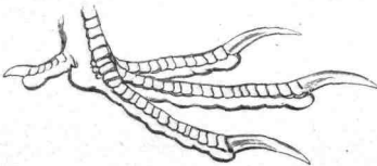
Fig. 25.—Foot of A. torqueola . 4.
