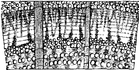
Fig. 46. Eichenholzquerschnitt. \frac{3}{1} .
