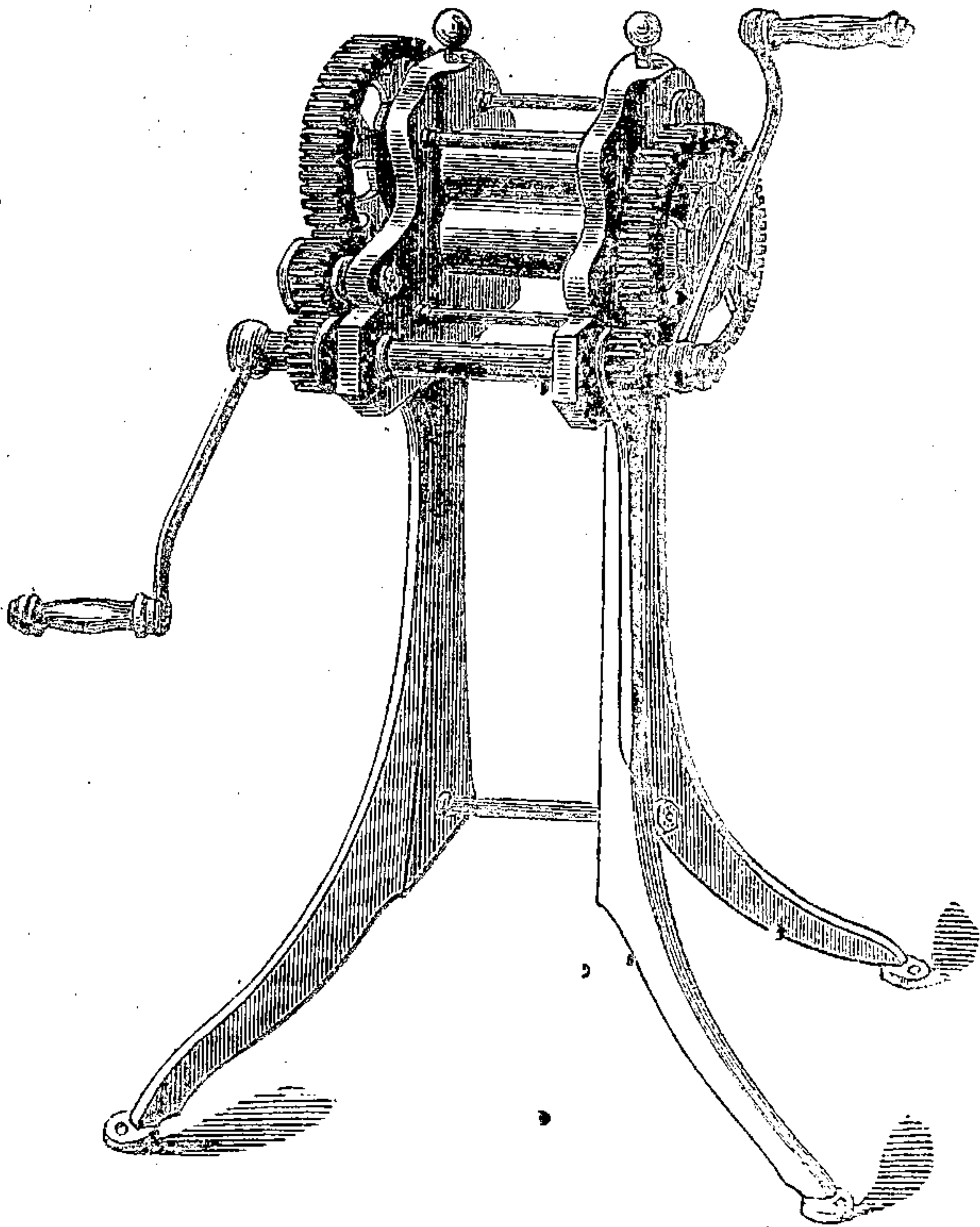
Fig. 25. Rollers for Gold.
