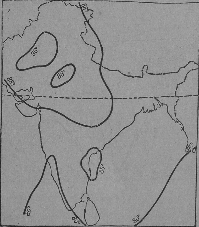
ஜூலை வெப்பநிலை
