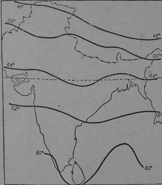
ஜனவரி வெப்பநிலை
