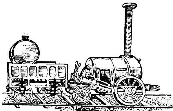
படம் 68. இராக்கெட் எஞ்சின்
