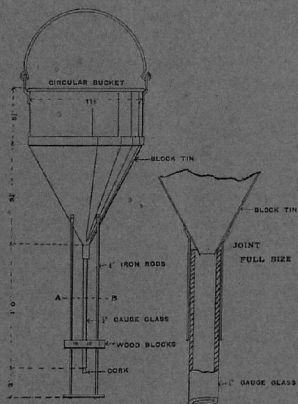
SECTION A.B.
