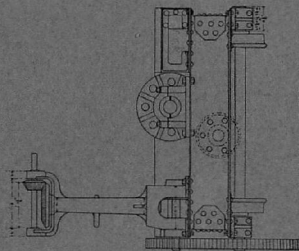
END ELEVATION
