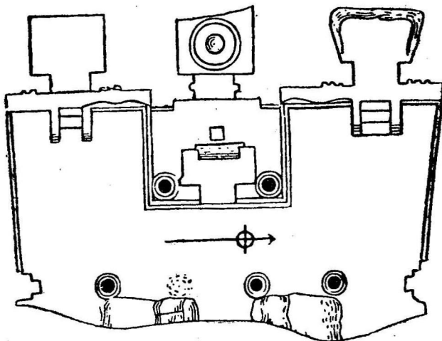
“மகிஷாசுர மண்டபம்” என்னும் கயிலாசநாதர் குகைக்கோயிலின் தரையமைப்புப் படம்
