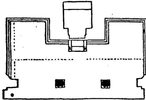
“வராக மண்டபம்” என்னும் குகைக்கோயிலின் தரையமைப்புப் படம்
