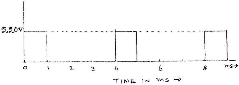
படம் 3 படம் 2இல் உள்ள இயக்கிக்கு SCR மூலம் அளிக்கப்படும் மின் அழுத்தம்.
