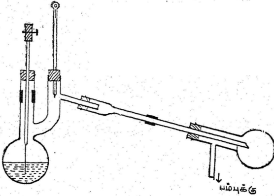
குறைந்த அழுத்தத்தில் காய்ச்சி வடித்தல்
