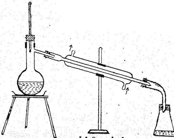
காய்ச்சி வடித்தல் படம்-6
