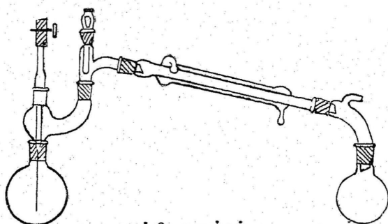
வெற்றிட வடித்தல் படம் - 19
