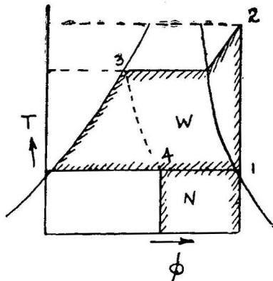
படம் 12 ஆவியிறுக்கச் சுழல் ( T - \phi வரைபடம்)
