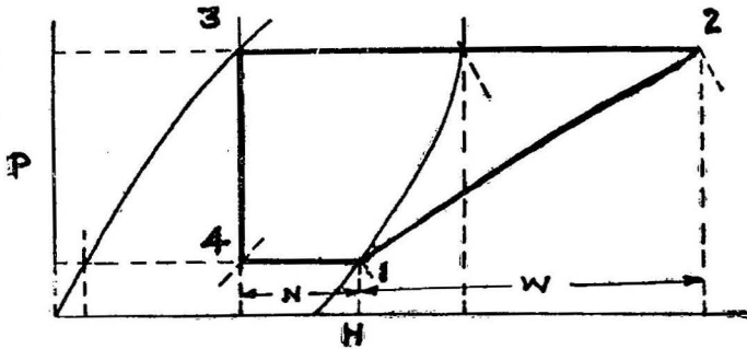
படம் 11 ஆவியிறுக்கச் சுழல்
