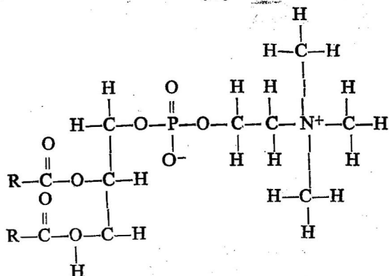
பாஸ்பாட்டிக் அமில கோலின் (லெசிதின்) [Phosphatidyl choline (Leeithin)] (உ)
