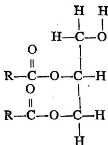
இரு கிளிசிரைடு (Diglyceride) (இ)
