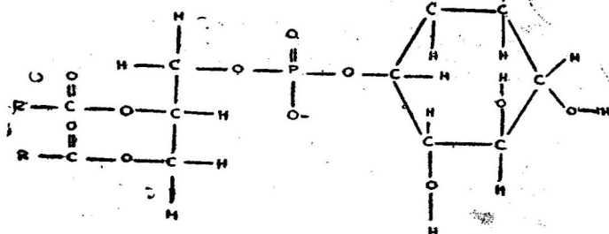
பாஸ்பாட்டிக் அமில இனோசிட்டைல் (PHOSPHATIDYL INOSITOL) (ஈ)
