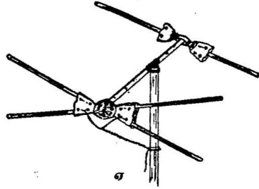
ஏ. கூம்பு வான்கம்பி.
