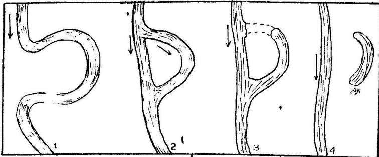
1. மியாண்டர் 2, 3, 4 குருட்டு ஆறு (OXBOW) 'அ' உண்டாகும் பல பழகளை விளக்கும் கின்றன.
