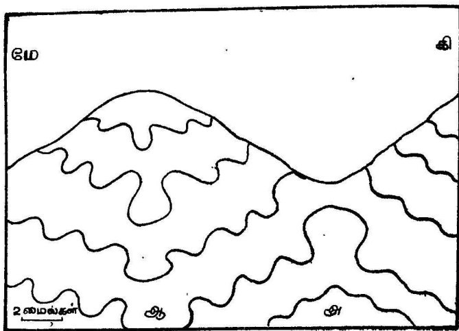
அ ஆன்டிகிளினோரியம் ஆ.சின் கிளினோரியம்
