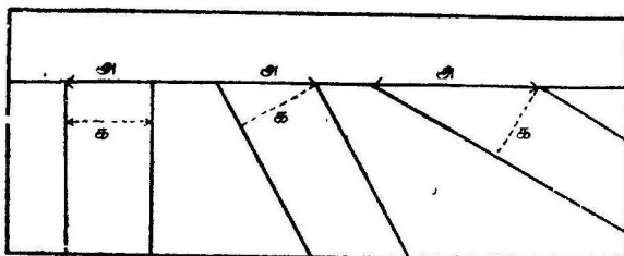
படம்-89 க. அடுக்குப் பாதையின் கனம் (THICKNESS) அ. பெளித் தெரிதலின் அகலம் (WIDTH)
