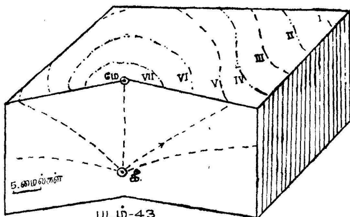
மே. மேல்மையம் (ENICENTER) கீ. கீழ்மையம் (FOWS) I-VII சம புவி அதிர்ச்சிக் கோடுகள்.
