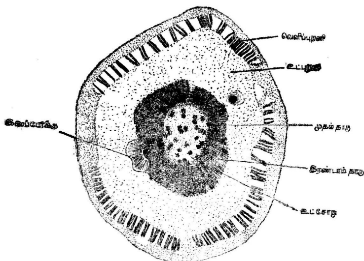
படம் 60. ஸ்டிரோமடெரிஸ்—தண்டின் குறுக்குவெட்டு
