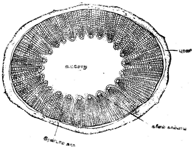
படம் 41. கலமைட்ஸ் தண்டின் குறுக்கு வெட்டு
