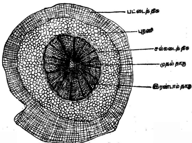
படம் 83. அமைலான்-வேரின் குறுக்கு வெட்டு
