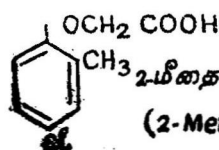
2,4-டை குளோரோபினொக்ஸி அசிடிக் அமிலம் '2,4-D' (2,4-Dichlorophenoxy acetic acid)
