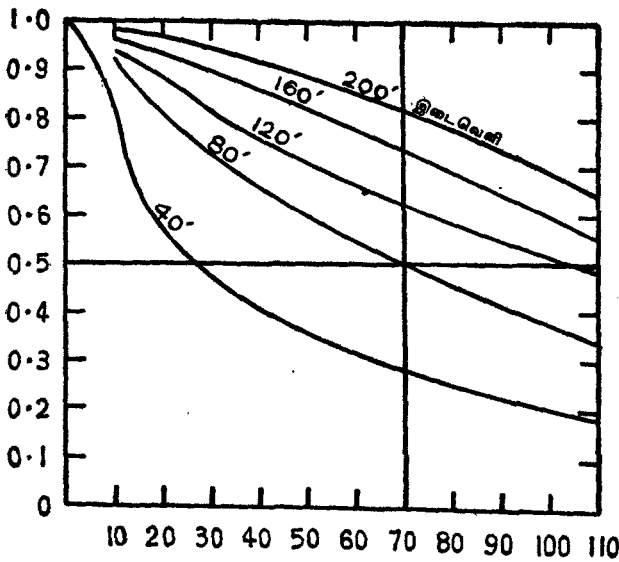
படம் 17. நீர்மூத்த ஊற்றுப் பகுதியில் வடிகால் கடை வெளியை நிர்ணயிக்க உதவும் வரை படம்
