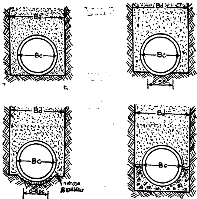
படம் 38. அகழியின் தளவகைகள்
