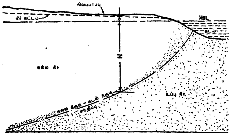
படம் 34. நல்ல நீர்-கடல்நீர் சந்திப்பு
