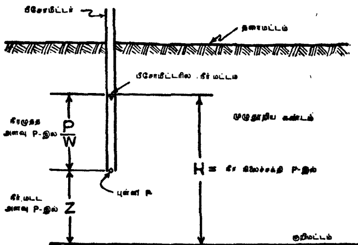
படம் 8. நீர்ச்சக்தியின் விளக்கம்
