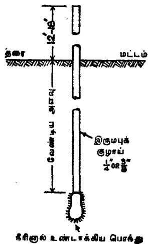
படம் 21. பீசோ மீட்டரும் அளவைக் கிணறும்
