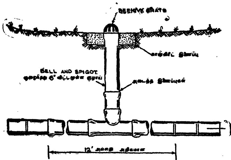
படம் 39. உள்போக்கியின் விளக்கம்
