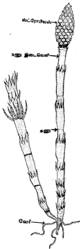
படம் 44 ஸ்ட்ரோபிலா:பைட்டின் அமைப்பு
