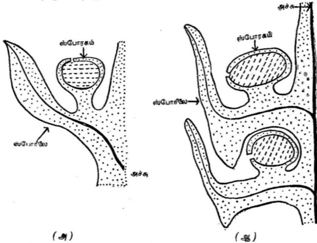
படம் 20 ஸ்போரகம் வெடித்தல்
