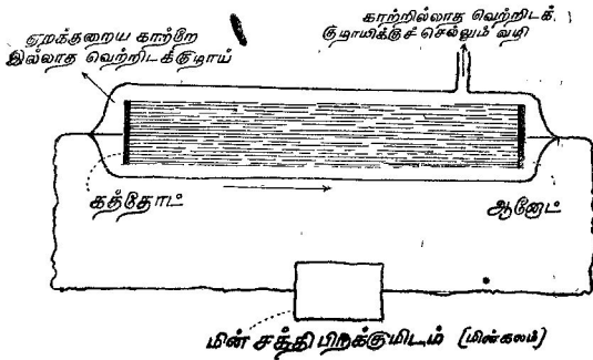
படப் 5. கீஸ்லர் குழாய்
