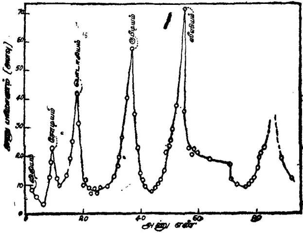
படம் 3. அணு எண்
