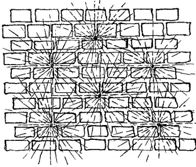
படம் 19. பலகணி அடுக்கு
