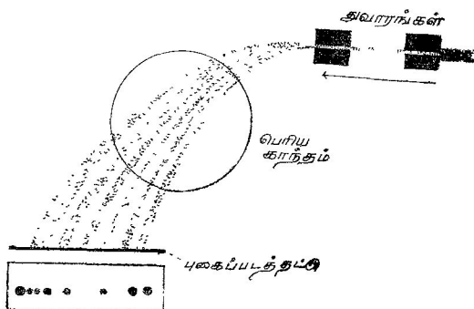
படம் 13. ஐஸ்டோப்புகளைப் பிரிக்கும் மாஸ் ஸ்பெக்ட்ரோ மீட்டர்
