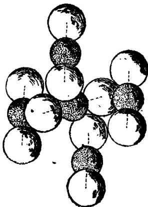
படம் 4. மொத்தையான (திடமான) கரியமிலவாயு அல்லது பனிக்கட்டியின் படிகம்
