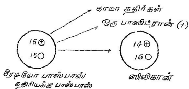
படம் 17. செயற்கைக் கதிரியக்கம்
