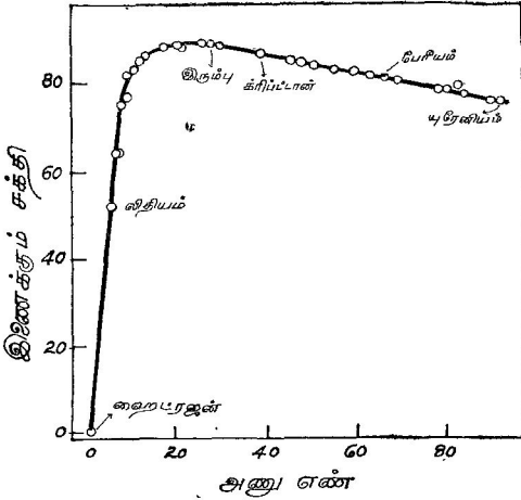
படம் 15 இணைக்கும் சக்தி (Packing Factor)
