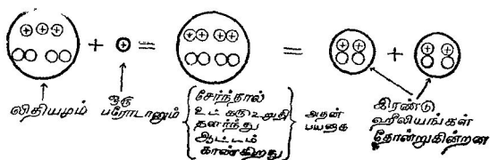
படம் 16. லிதியம் சிதைவு
