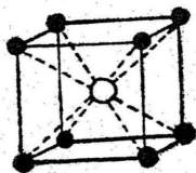
CsCl
