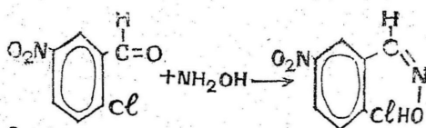
2-குளோரோ-5-நைட்ரோ பென்சால் மூலஹைடு
