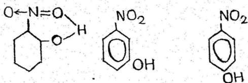
o-நைட்ரோபீனால் m-நைட்ரோபீனால் p-நைட்ரோபீனால்
