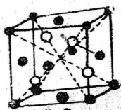
ZnS சங்கப் பிளாஸ்ட்
