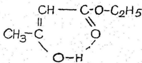
ஈதைல் அசெட்டேட் அசெட்டேட்
