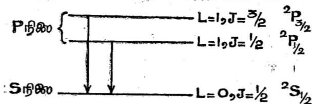
சோடியம் D வரிகளின் நுண்ணமைப்பு
