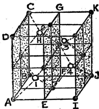
●-Zn ○-S
