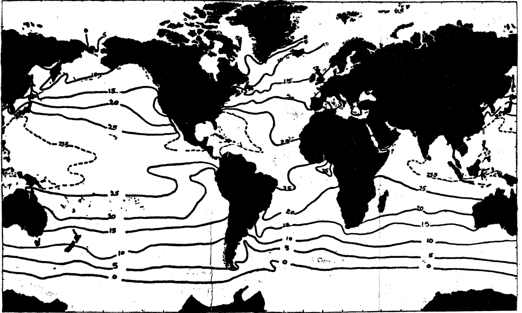
படம் 2.5. சமூக்திர மேல்தள வெப்பநிலை (ஆண்டு) பரவல்.
